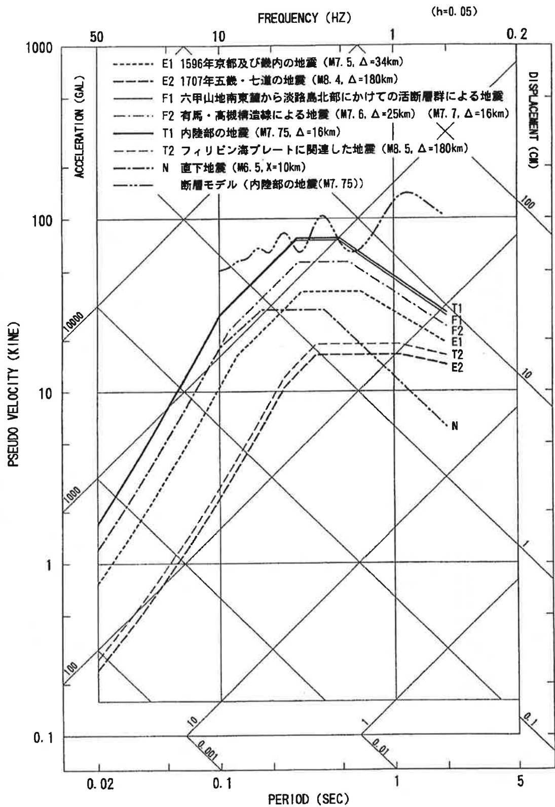
第5-4図 神戸において想定される地震動の応答スペクトル
