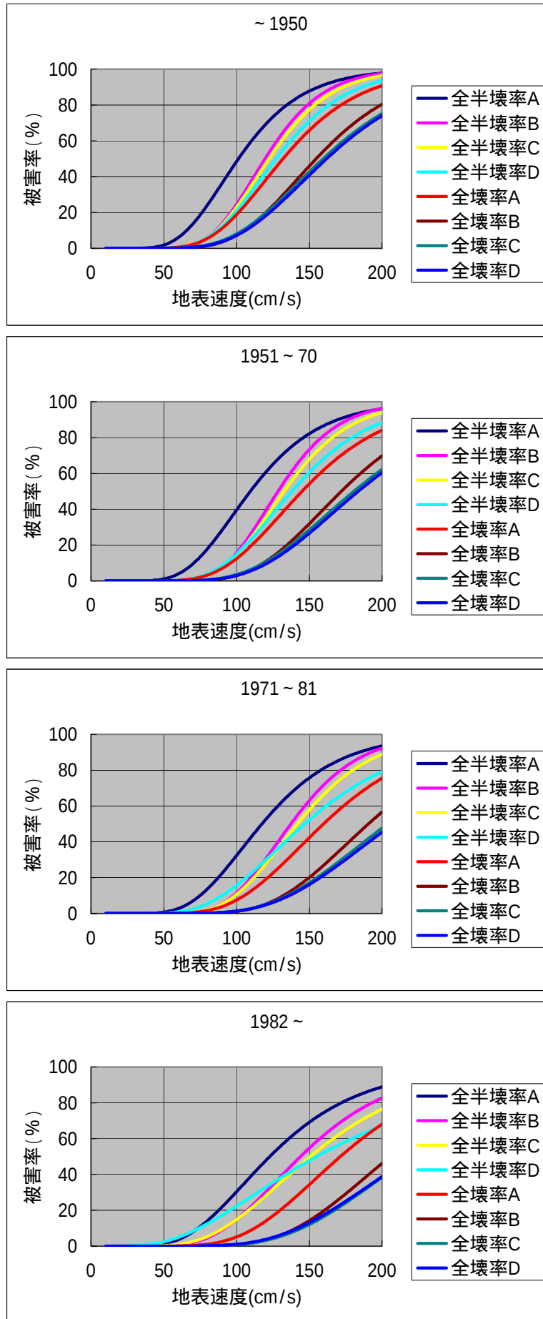
図 4-1-3(2) 木造建物の被害率曲線（内陸型）
