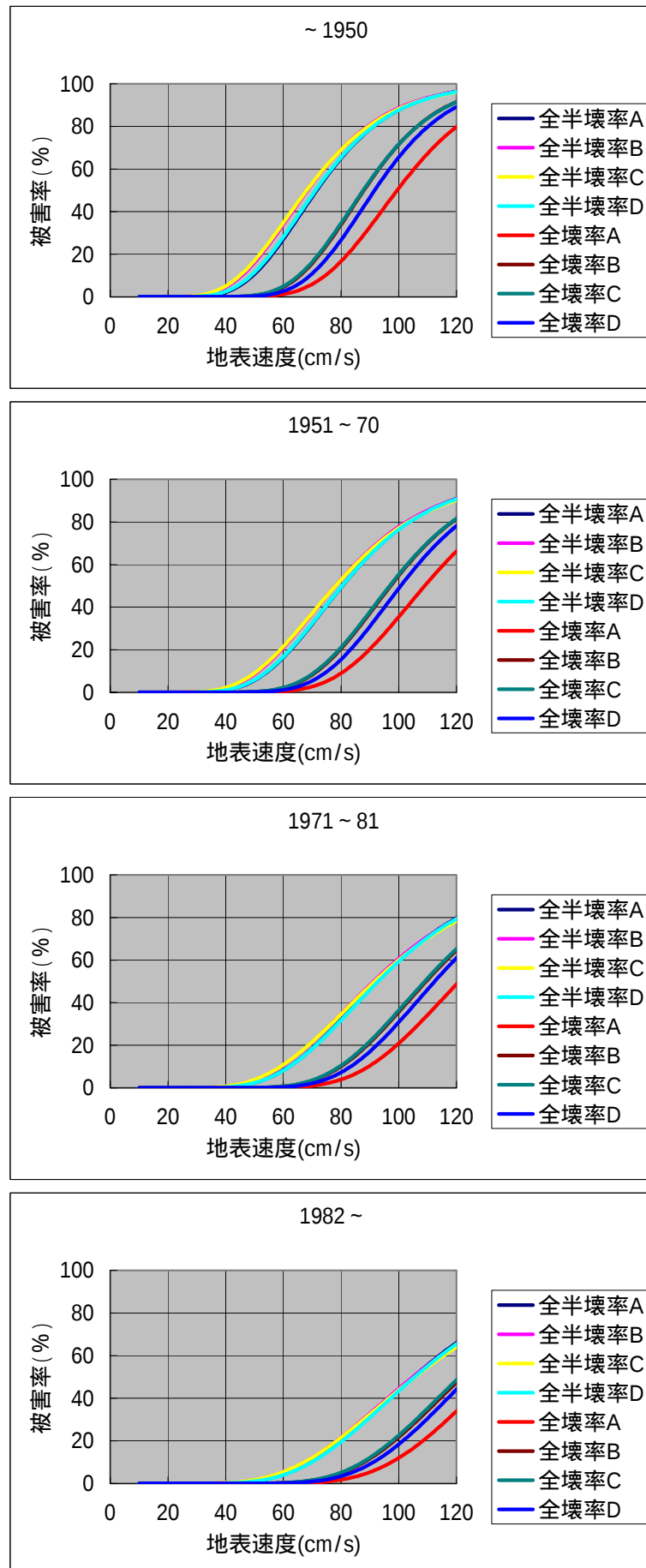
図 4-1-3(1) 木造建物の被害率曲線（海洋型） A、B、C、Dは地盤タイプを示す。
