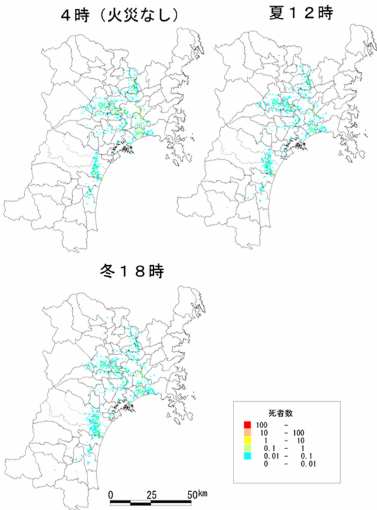
図 4-3-6 死者数分布図（宮城県沖地震(単独)）
