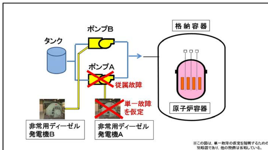
図2 単一故障しても、安全機能が維持される例
