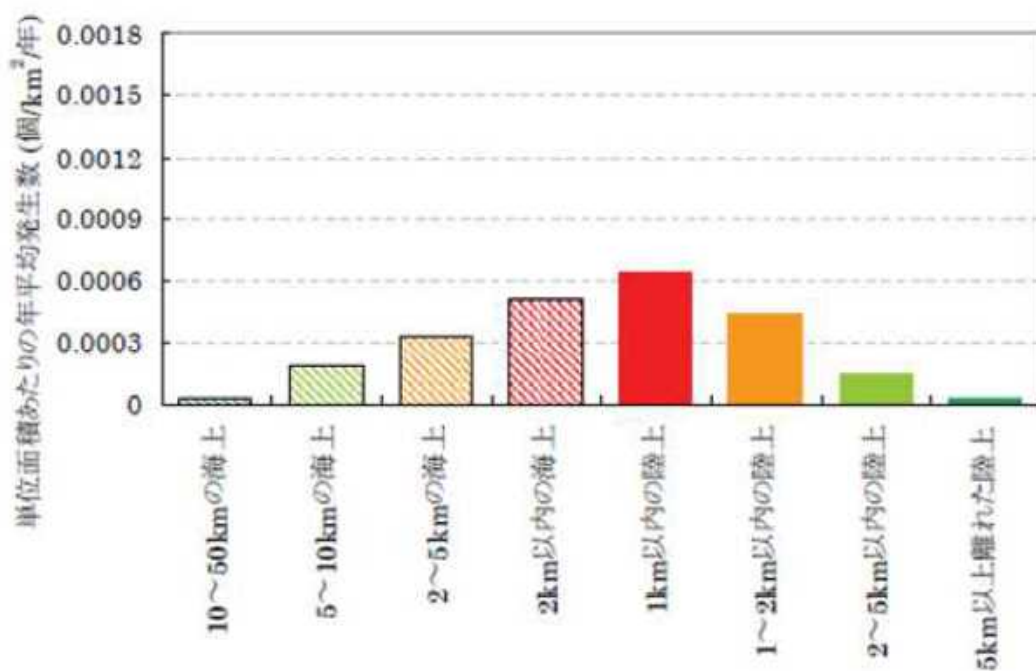
図3 日本の海岸線付近における竜巻の発生状況 *1 （1961～2009 年 12 月、規模：F 0
