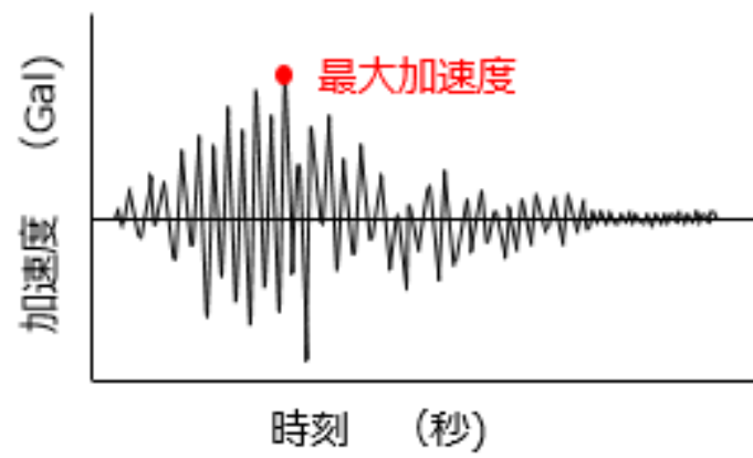
図 4 基準地震動の概要
