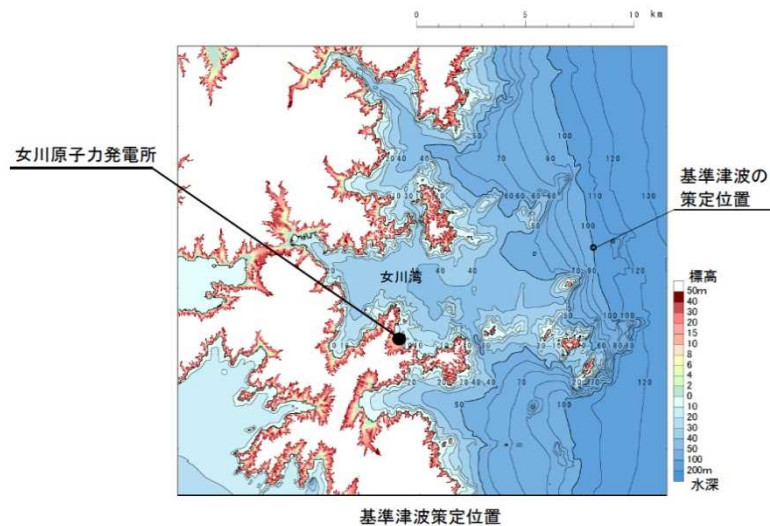
図7 基準津波の策定位置（例）
