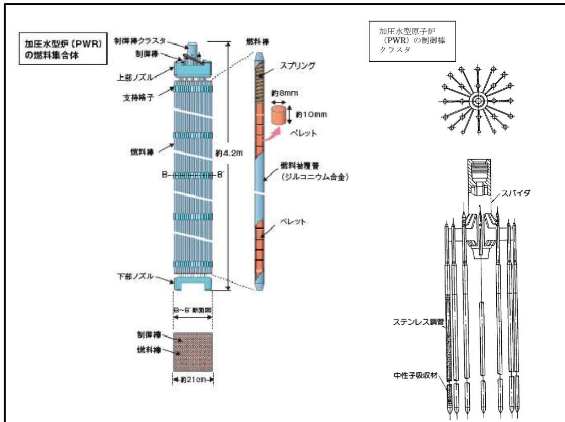
図 5 P W R の 燃 料 集 合 体 及 び 制 御 棒
