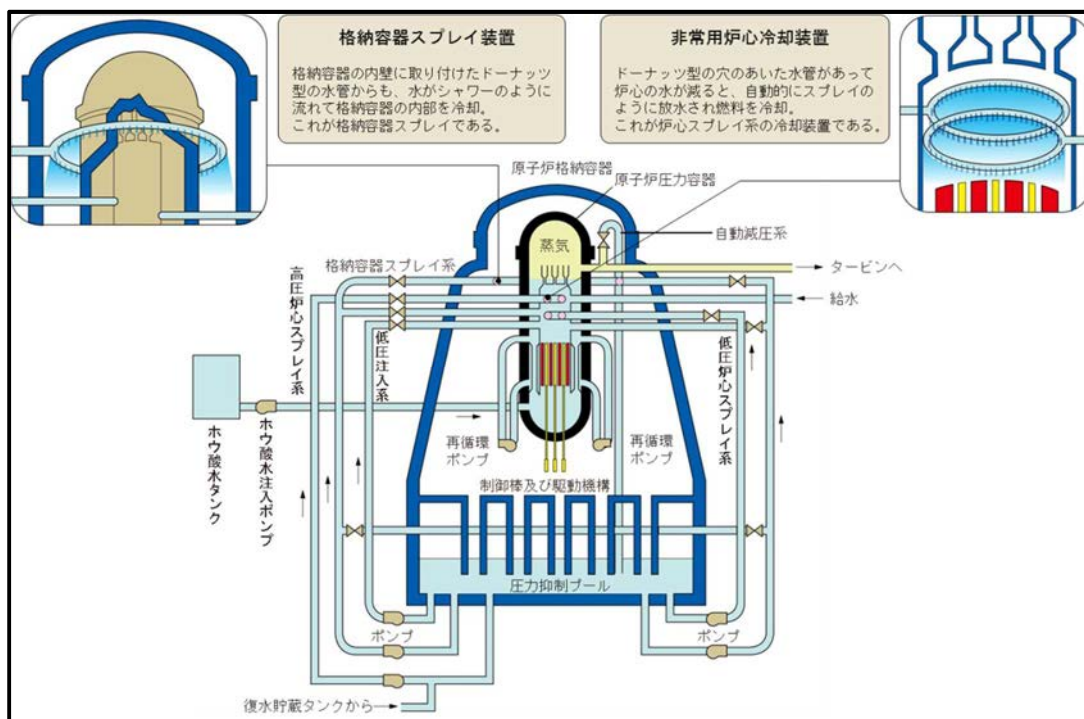
図 2 BWR の非常用炉心冷却装置等の例 (出典：日本原子力文化財団，原子力・エネルギー図面集 2015)
