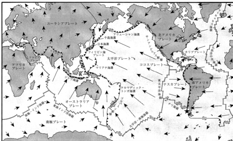
図1 世界のプレート境界
