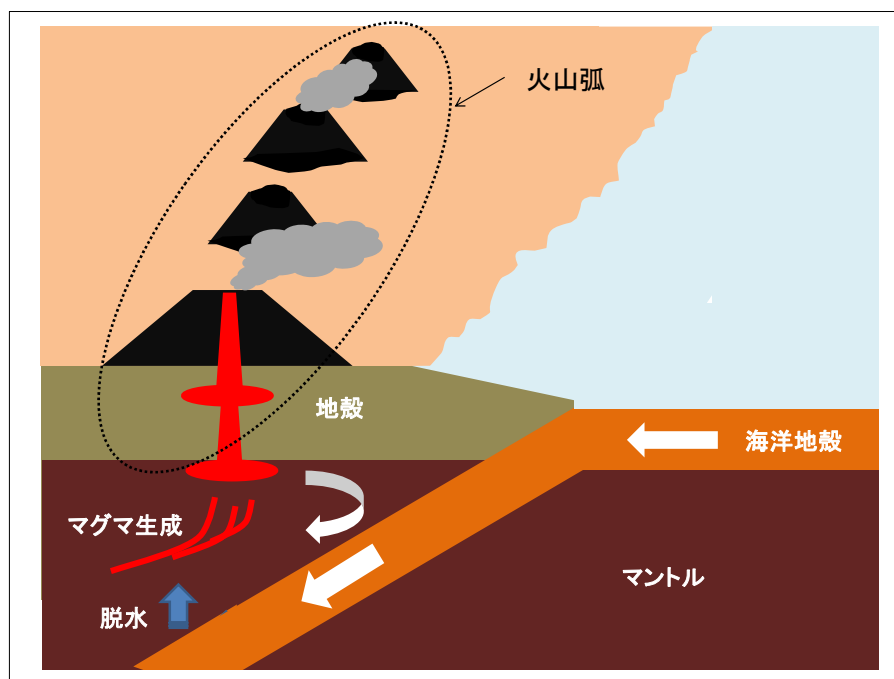
図２ 火山活動の仕組み
