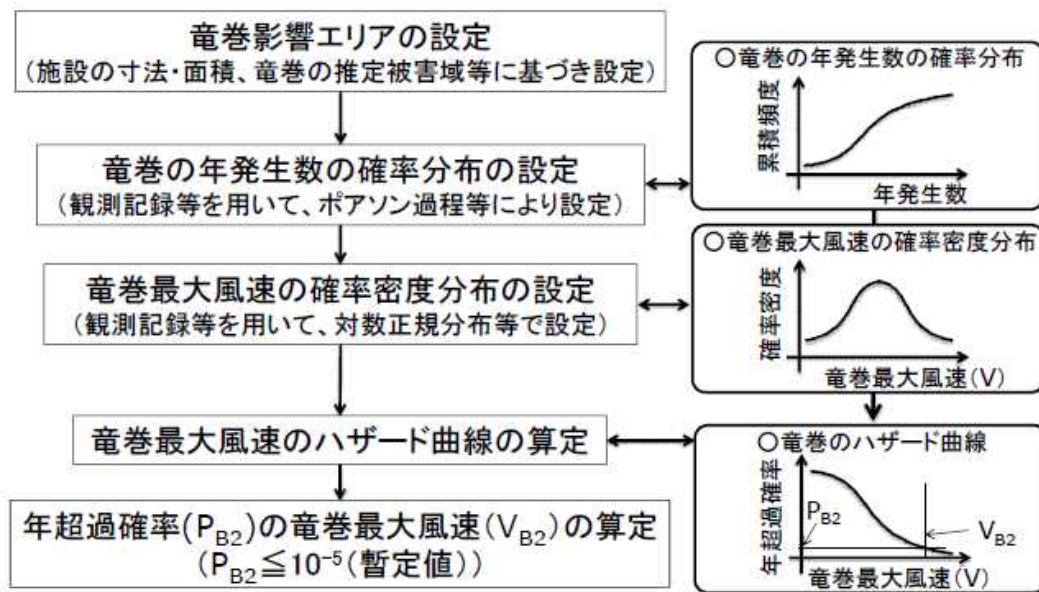
図4 竜巻最大風速のハザード曲線による最大風速 ( V_{B2} ) の算定フロー
