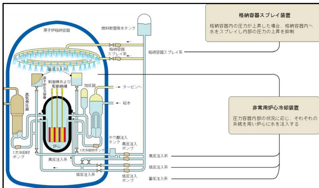
図 3 PWR の非常用炉心冷却装置等の例 (出典：日本原子力文化財団，原子力・エネルギー図面集 2015)
