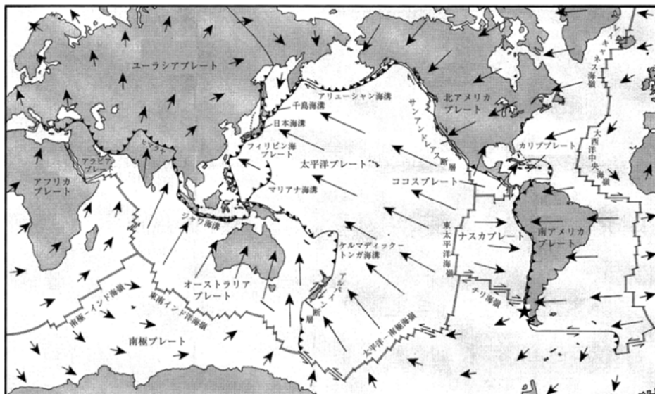
図1 世界のプレート境界
