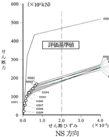
図-5-③ 原子炉建屋の最大応答せん断ひずみ
