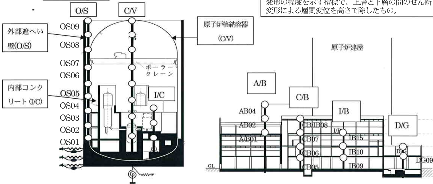
図-5-① 原子炉建屋の解析モデルの概念図
