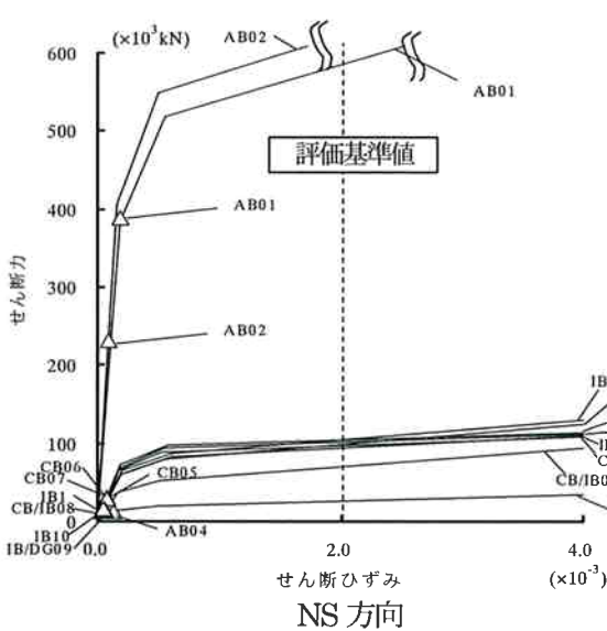
図-5-④ 原子炉補助建屋の最大応答せん断ひずみ
