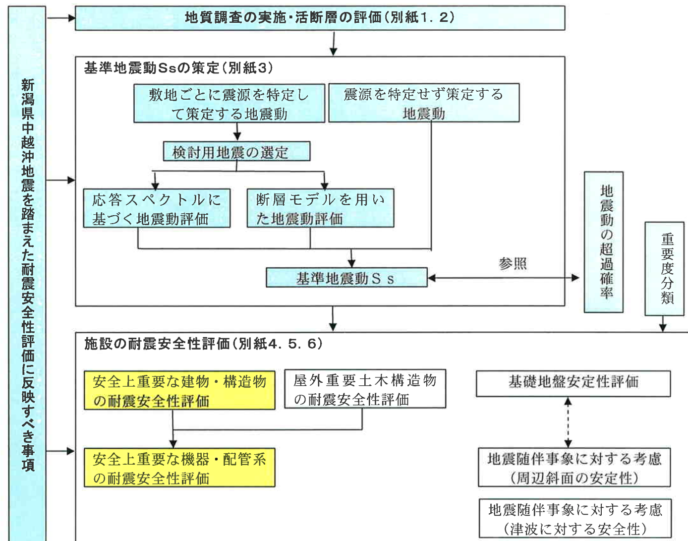
図-1-① 耐震安全性評価の流れ
