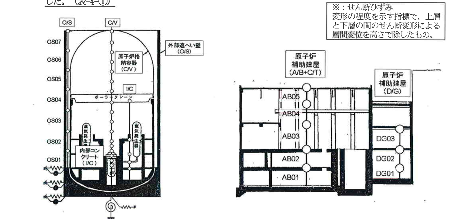
図-4-① 原子炉建屋の解析モデルの概念図
