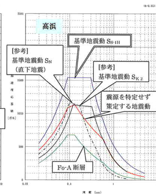
図-3-② 応答スペクトルに基づく地震動評価（高浜）
