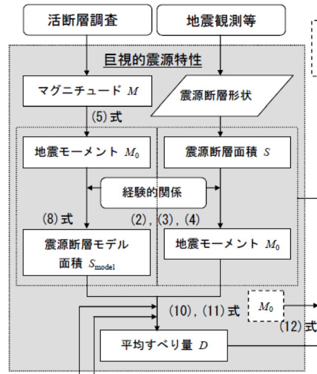
付図2 活断層で発生する地震の震源特性パラメータ設定の全体の流れ
