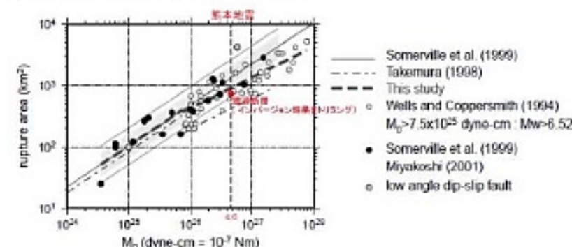
図1 入倉・三宅式と熊本地震の比較
