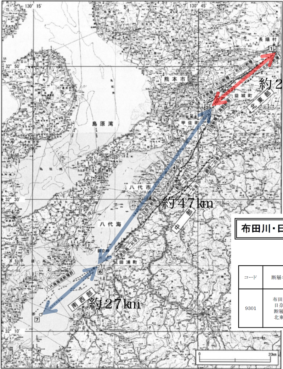
図2 布田川・日奈久断層帯の活断層位置と調査地点
