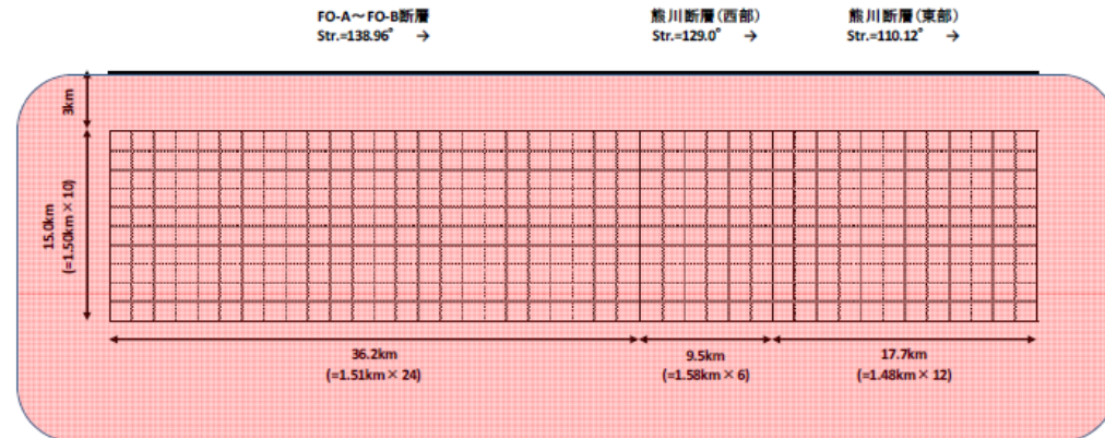
武村式に置き換えたアスペリティ(赤色)のイメージ
