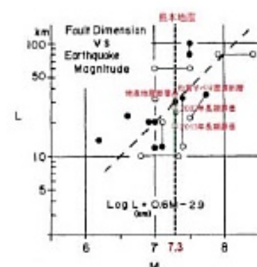
図2 松田式と熊本地震の比較
