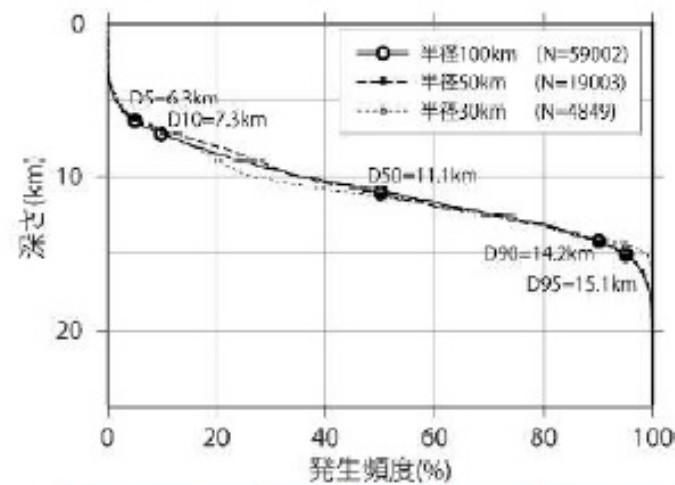
気象庁一元化震源 (2000年1月～2012年12月)
