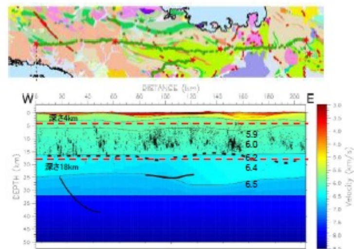
図 10 藤橋—上郡測線の地震波速度構造に、測線周辺の震源分布と反射法解析によって見出された反射面を重ねた。
