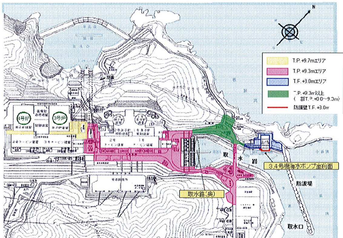
【図表 2 津波水位の評価点】
