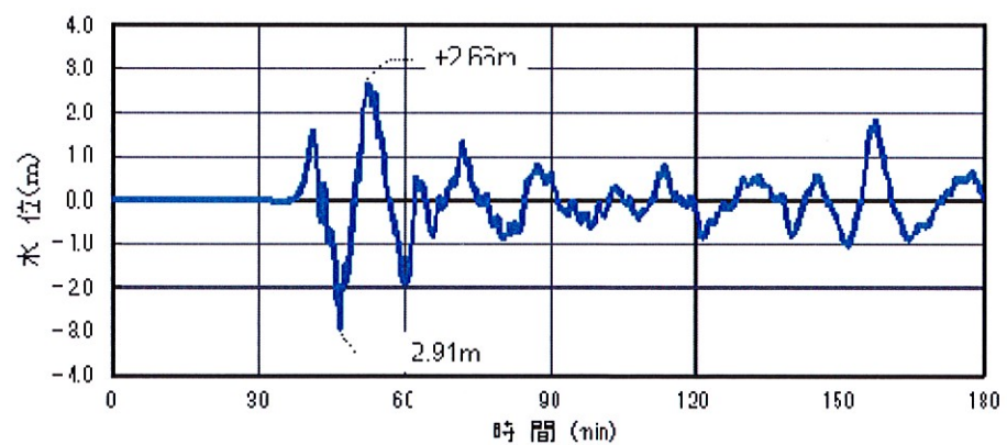
【図表 1 5 基準津波 1 の時刻歴波形】
