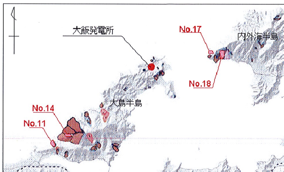
【図表 9 陸上地すべり地形の抽出結果】
