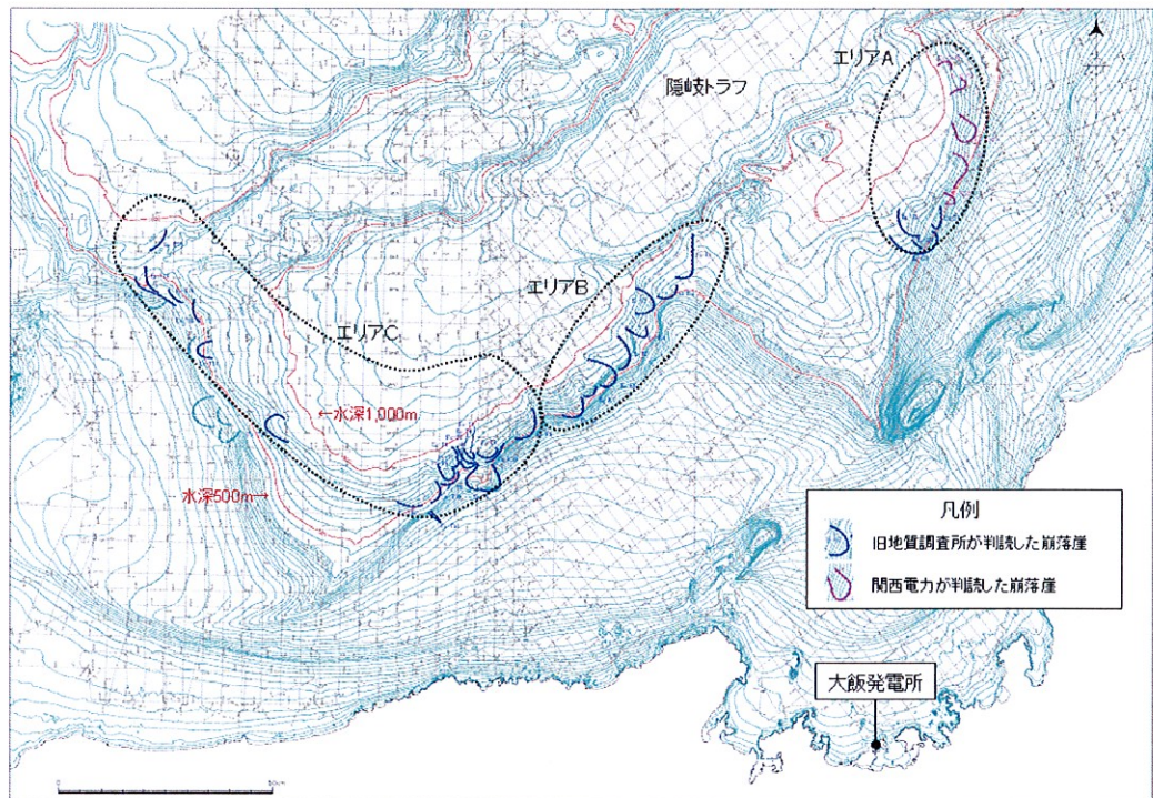
【図表 7 検討対象とした海底地すべり地形】
