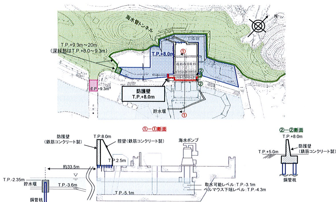
【図表 1 8 本件発電所海水ポンプ室周辺地盤及び防護壁並びに貯水堰】
