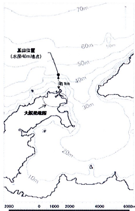
【図表 1 4 基準津波の策定位置】
