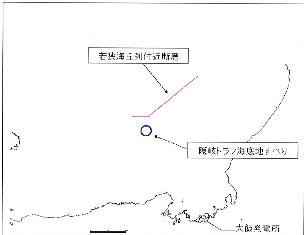
【図表13 基準津波の波源位置】
