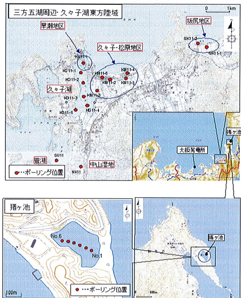
【図表 3 津波堆積物調査位置】
