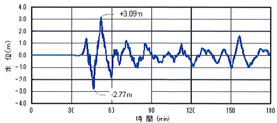
【図表 1 6 基準津波 2 の時刻歴波形】
